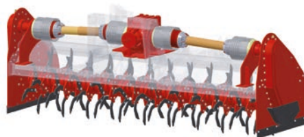
MONO rotore fresante MONO tilling rotor
